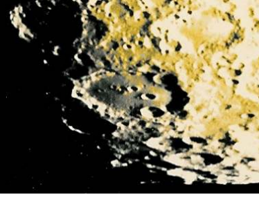
Abb. 45-9: Ringwall Clavius dicht an der Lichtgrenze mit deutlichem Schatten, aufgenommen mit einem 15 cm Refraktor
