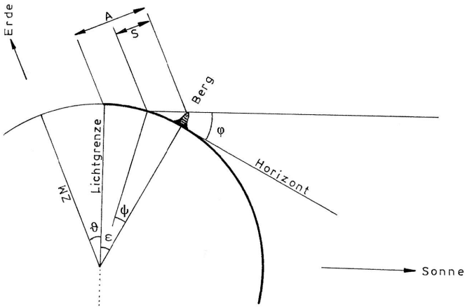
Abb. 45-11: Winkel und Strecken zur Bestimmung der Höhen von Mondbergen
