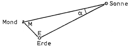
Abb. 45-10: Dreieck Sonne-Erde-Mond
